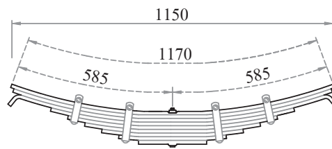
แหวนช่วงกลาง 3 เผลา ปลายงอ 2 ด้าน
