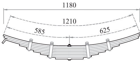
แหวนหน้า/หลัง ปลายงอด้านเดียว
