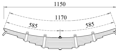
แหนบช่วงกลาง 3 เฟลา ปลายงอ 2 ด้าน
