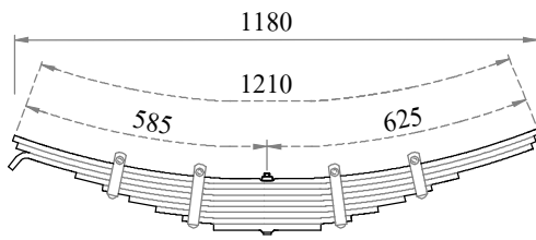
แหนบหน้า/หลัง ปลายงอด้านเดียว
