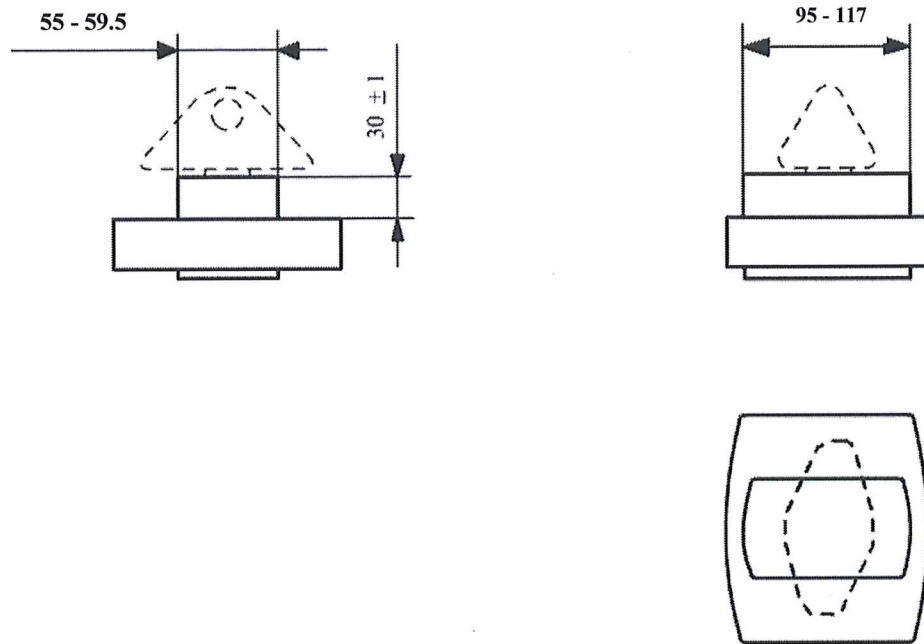
ภาพที่ ๓ ขนาดของปลอกจับ (หน่วย : มิลลิเมตร)
