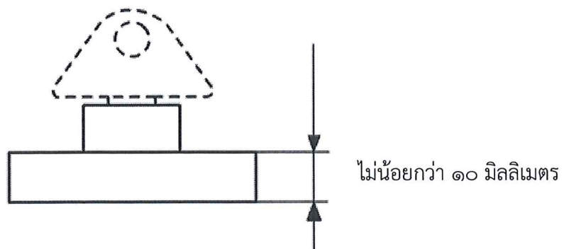
ภาพที่ ๒ ขนาดของแผ่นรองรับมุมตู้บรรจุทุกสินค้า (หน่วย : มิลลิเมตร)
