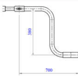
12-3220 ชุดมือหมุนขาค้ำยัน ขนาด 32 x 750 x 380 มม.
