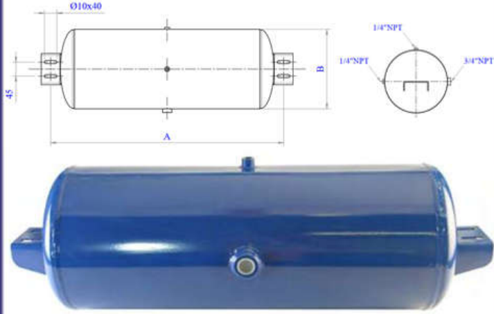
ขนาดสัดส่วนถังลมเหล็ก
