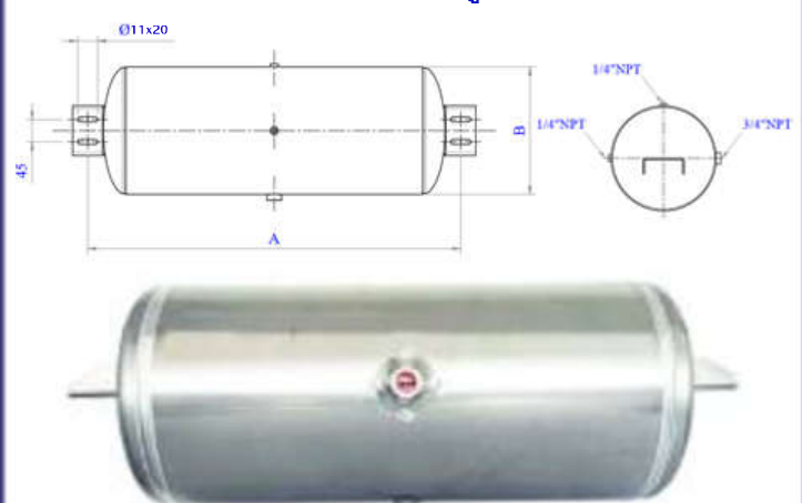
ขนาดสัดส่วนถังลมอลูมิเนียม
